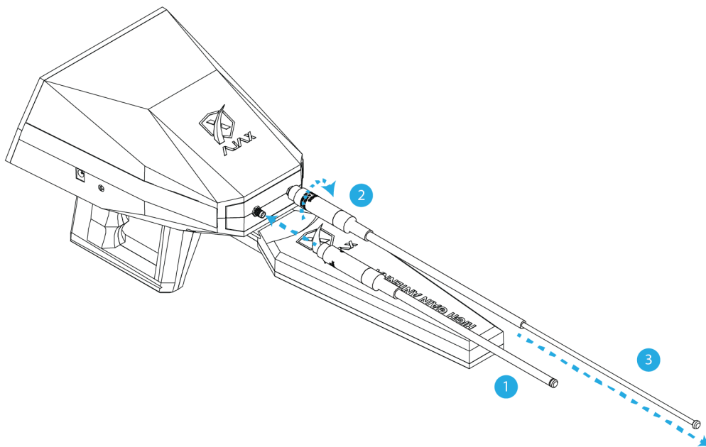
figure 6 - Montaje de Antena de Seguimiento
